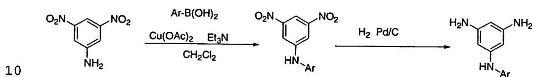
Scheme II-A
